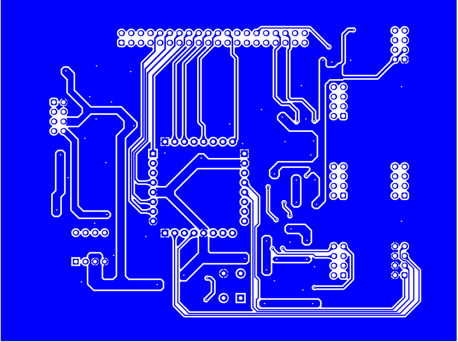
Bottom Layer (Scale 1:1)
